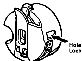
Special bobbin case Spezial-Spulenkapsel
