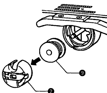
Special bobbin case Spezial-Spulenkapsel
